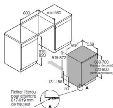
Dimensions d'encastrement
